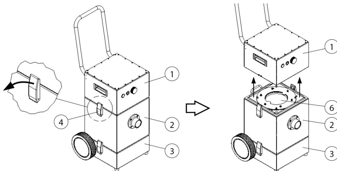
Fig. 9: Rengjøre filterpatronen
