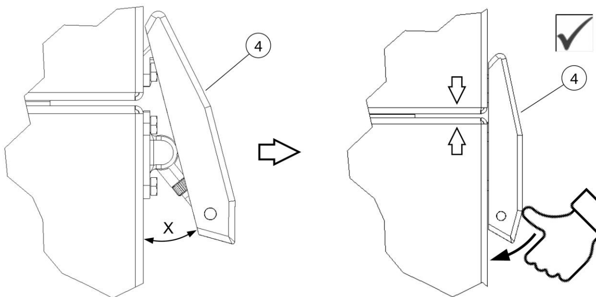
Fig. 12: Etterjustere strammelås
