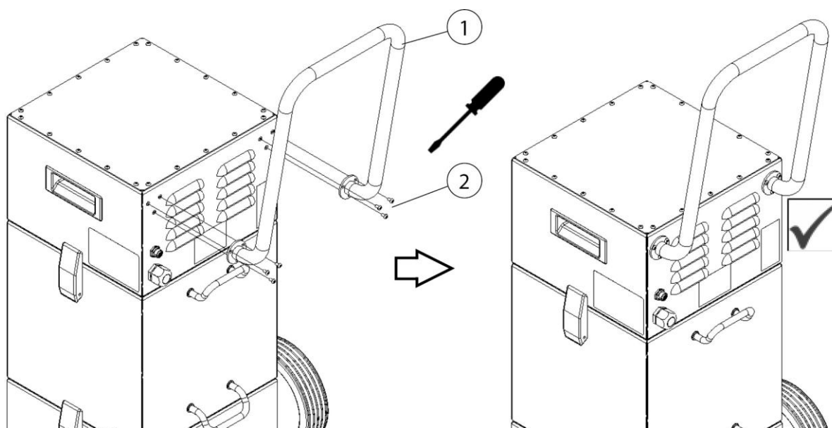
Fig. 3: Montere skyvehåndtak
