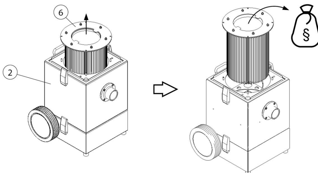
Fig. 15: Kast filterpatronen
