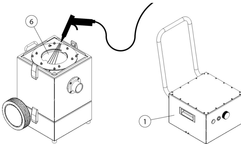
Fig. 10: Rengjøre filterpatronen
