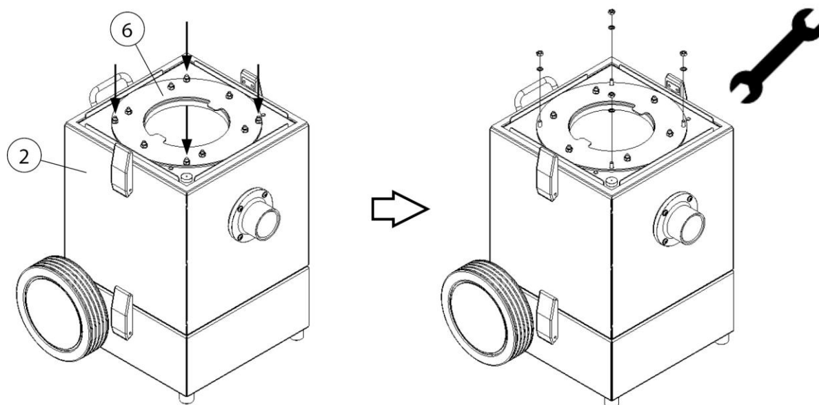
Fig. 14: Demontere filterpatronen
