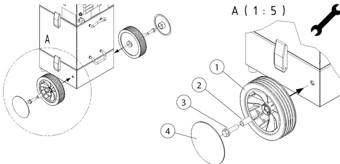
Fig. 2: Montering av bakhjulene
