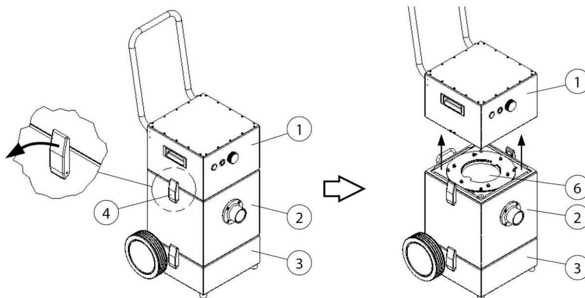
Fig. 13: Tilgang til hovedfilteret
