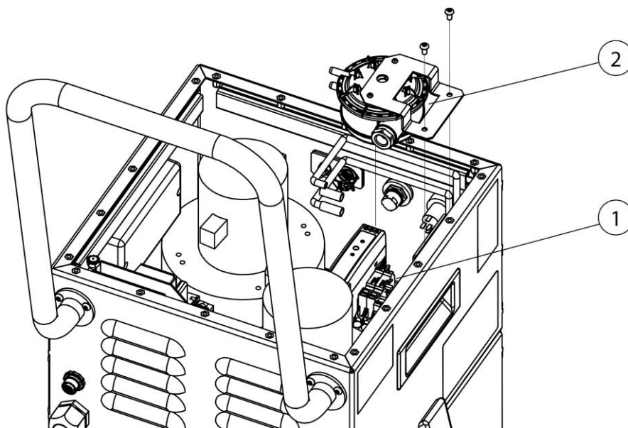
Fig. 16: Tilgang til sikringene
