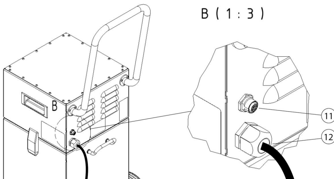
Fig. 5: Start/stopp-automatikk
