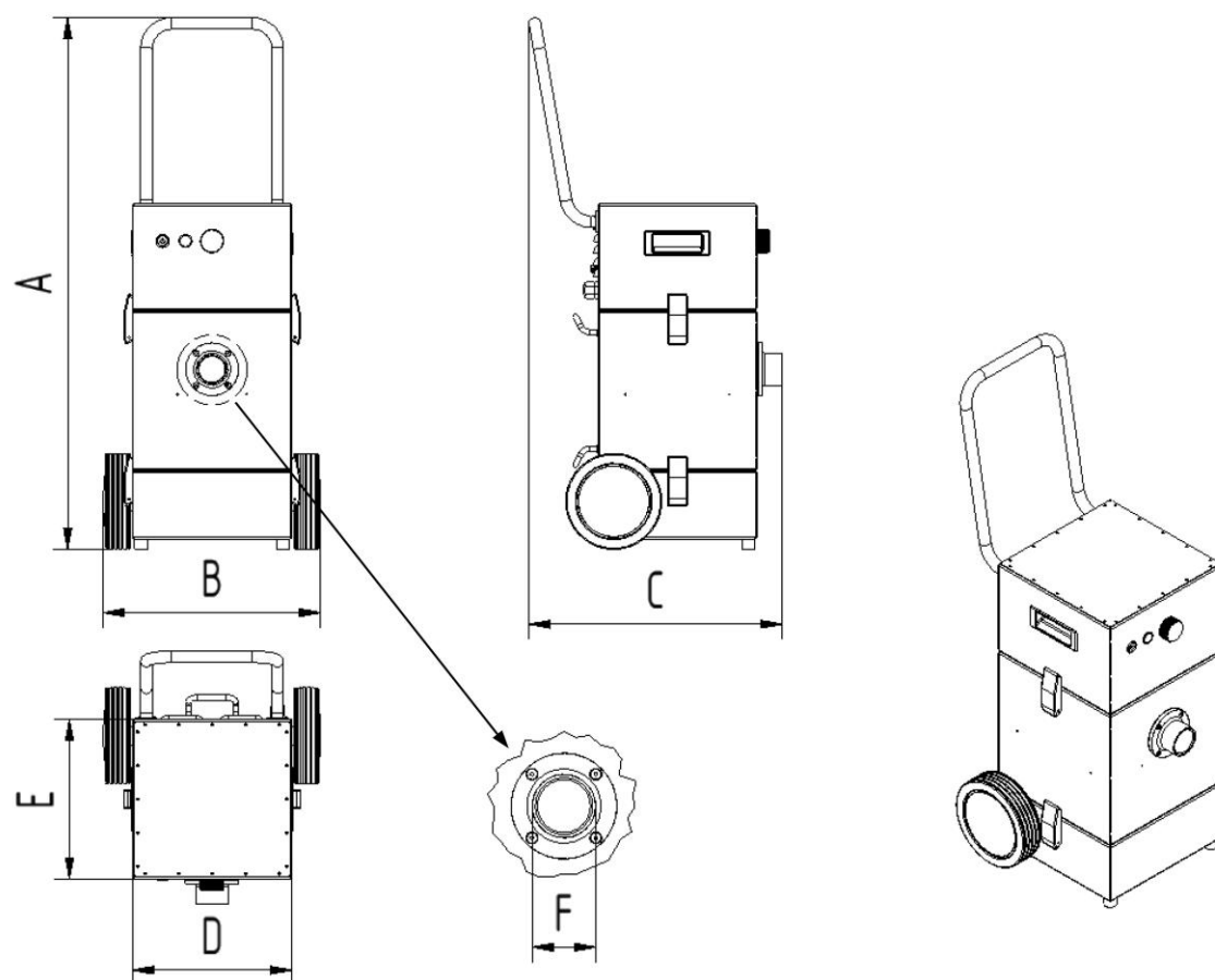
Fig. 17: Målskisse
