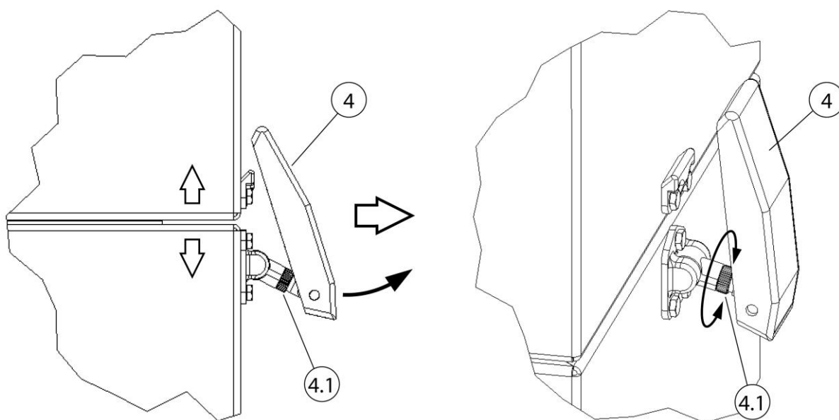
Fig. 11: Etterjustere strammelås
