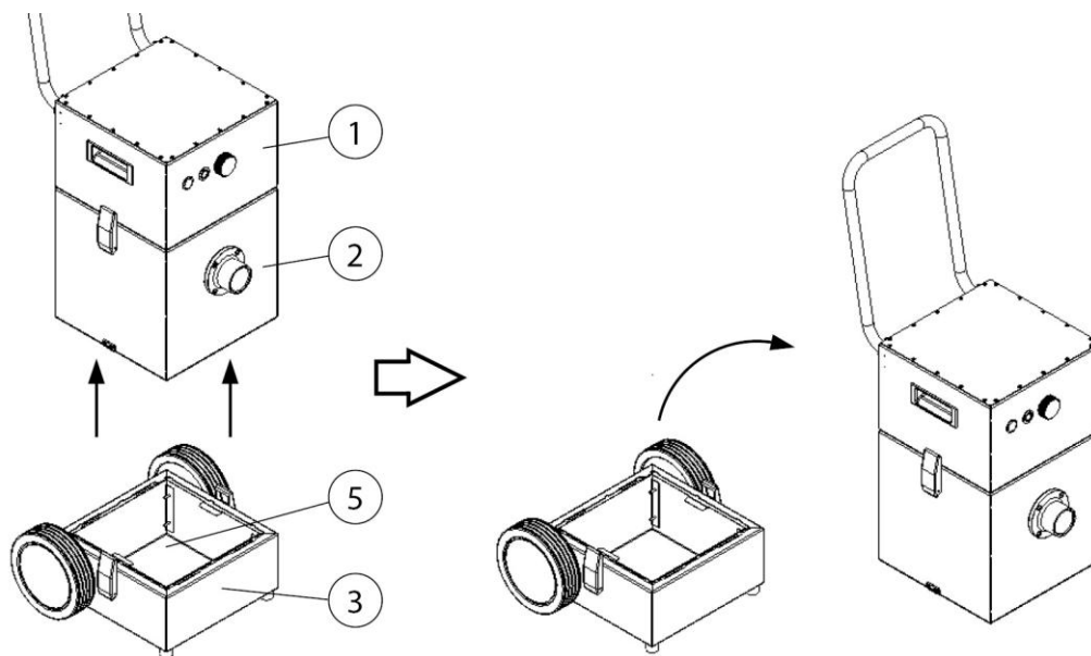
Fig. 7: Løfte filterenheten
