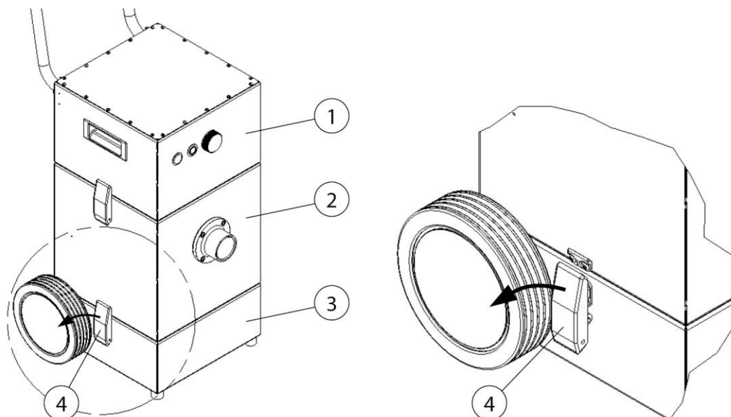
Fig. 6: Skifte støvsamlebøtte
