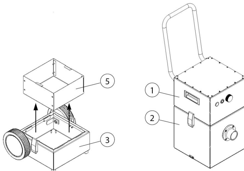
Fig. 8: Fjerne støvbeholder
